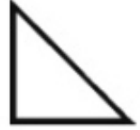
164. Triangle ತ್ರಿಕೋನ
